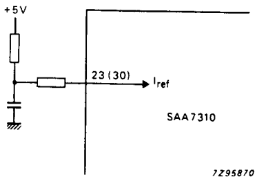
Fig. 13 I_{ref} circuit.
